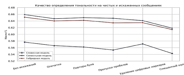
Рис. 1. Изменение Macro-F1 при разных видах текстового шума
